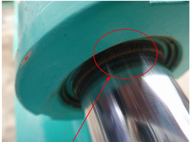
アームシリンダーパッキンひび割れ有り。
