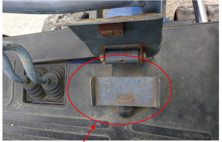
スイングペダル固着ぎみ。
